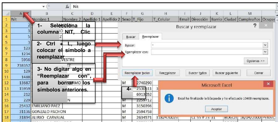
Figura 24. Herramienta reemplazar
